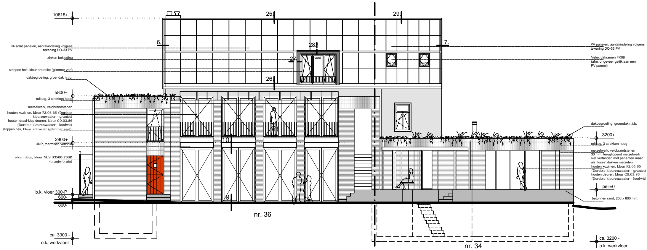
OOSTGEVEL - loodrecht aanzicht hoofdgebouw
