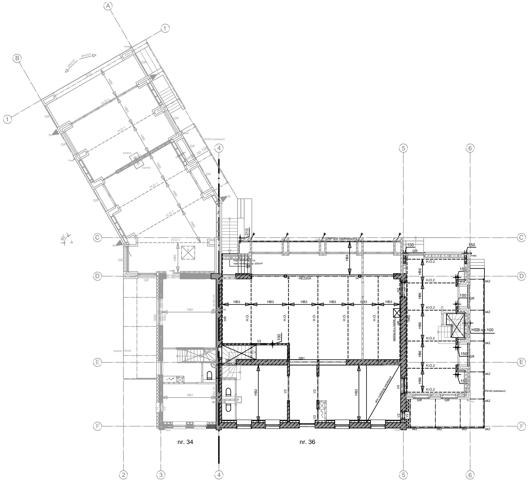
EERSTE VERDIEPING VLOEREN + DAKBALKLAAG
