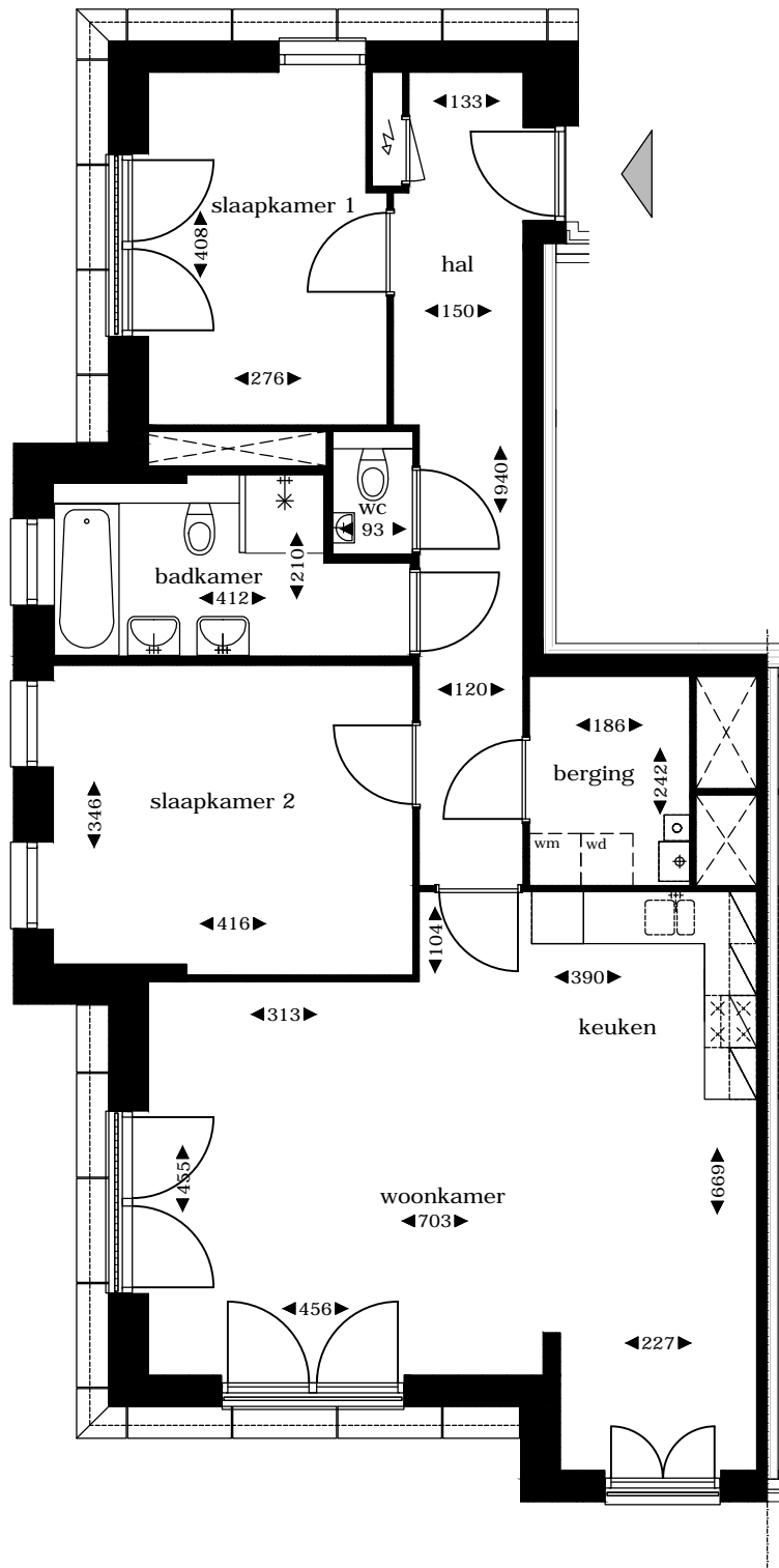
woningtype C2
