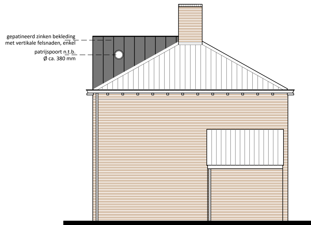
OOST-GEVEL NIEUW
