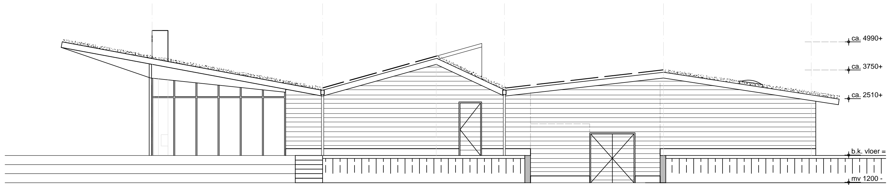
OOSTGEVEL
