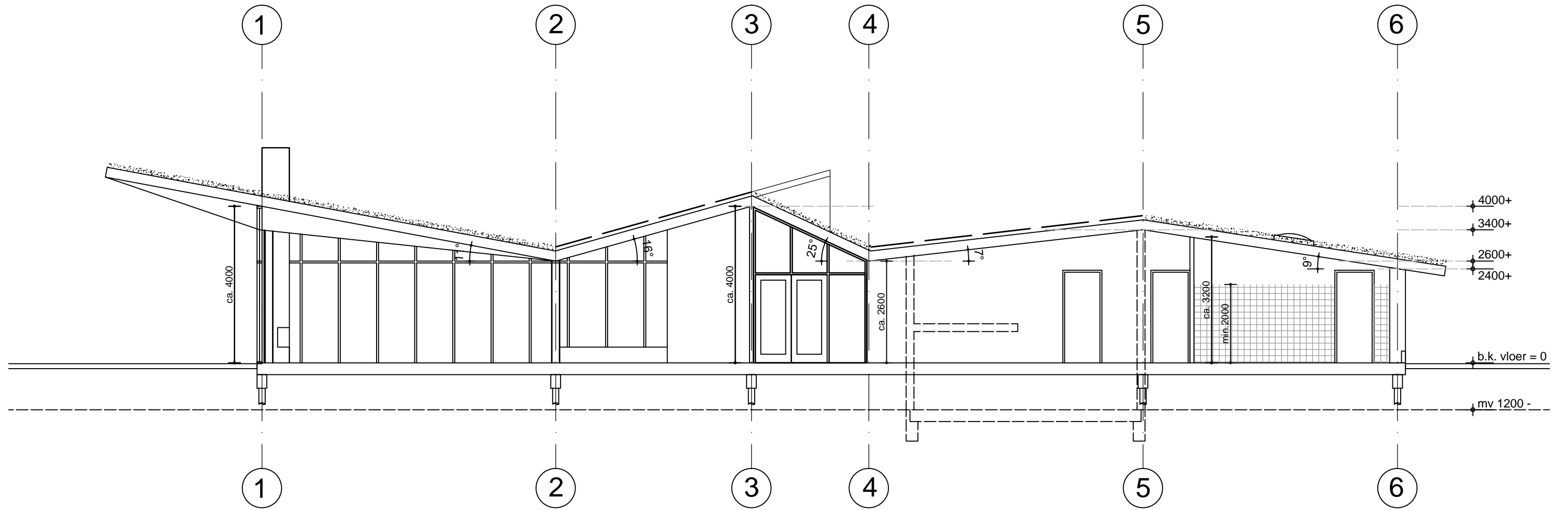
DOORSNEDE A-A
