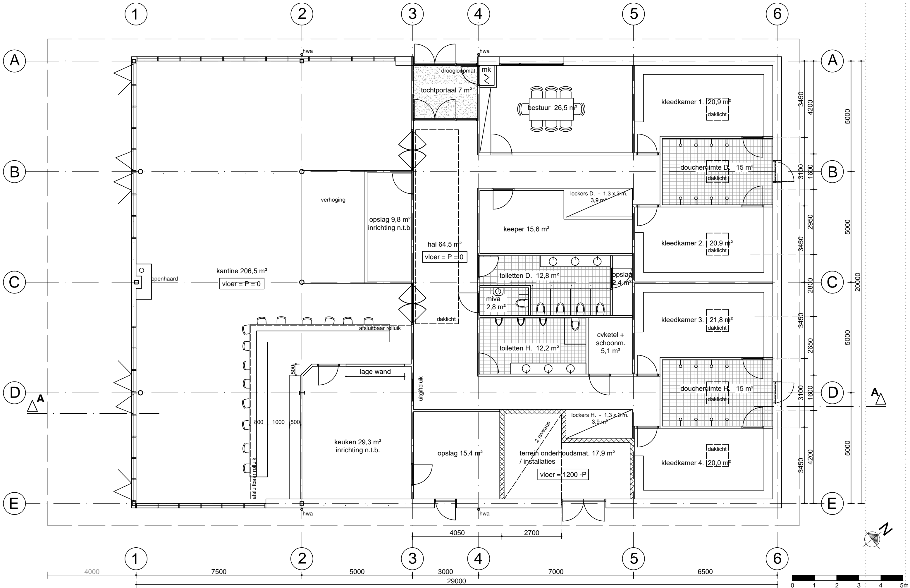
PLATTEGROND
